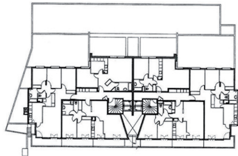
Plan d'étage courant.
